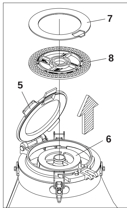
Detalle "F"
