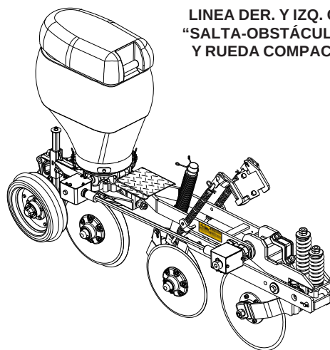
LINEA DER. Y IZQ. CON Y SIN SISTEMA "SALTA-OBSTÁCULO" C/ PUNTA SURCADORA Y RUEDA COMPACTADORA DE HIERRO
