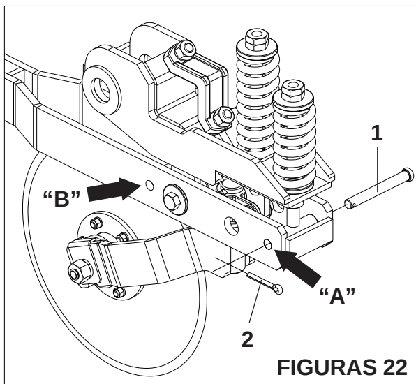
Sistema “Salta-Obstáculo” listo para el trabajo
