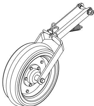
CARRITORUEDA COMPACTADORA CONVEXA
