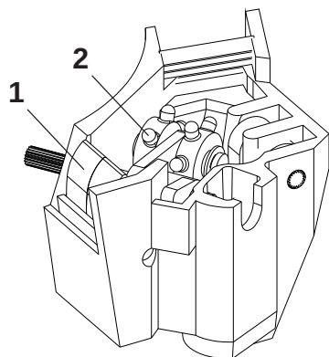
Caja Dosificadora de Semilla
