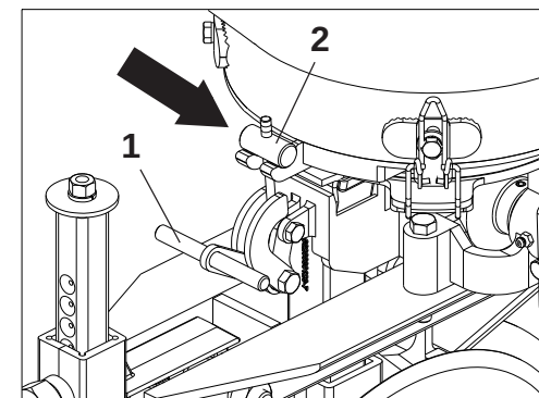
Detalle "A"
