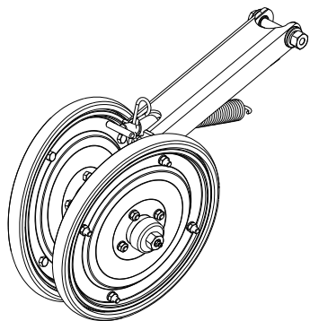
CARRITORUEDA COMPACTADORA CONVEXA
