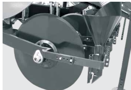
Sistema aplicador conjugado de adubo. Aplication System of conjugated fertilizer. Sistema aplicador conjugado de abono.
