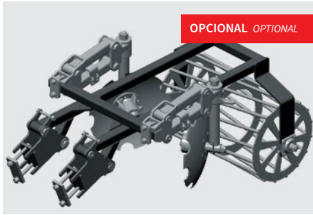
Conjunto pantográfico para cultivador (cana crua). Cultivator pantographic set (sugar cane). Kit paralelogramo para cultivador (caña cruda).
