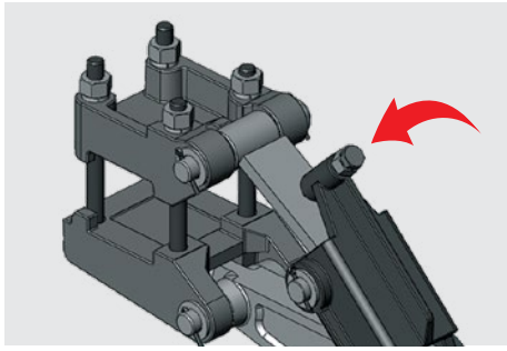
Ajuste de pressão do desarme. Reset pressure adjust. Ajuste de presión del sistema.
