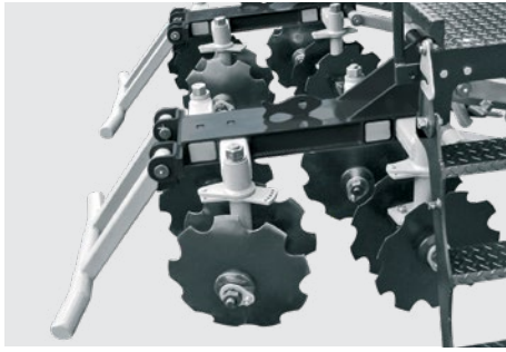
Grade em sistema pantográfico (cana queimada). Parallel flotation system (burned sugar cane). Rastra armada em sistema pantografico (caña queimada).
