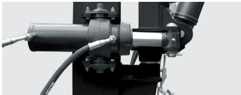
Pistão de giro da torre (GTG e GTG-RO 1200). Arm controlled by hydraulic system (GTG and GTG-RO 1200). Pistón de giro de la torre (GTG y GTG-RO 1200).
