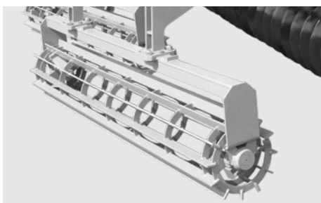
Rolo destorroador tem a função de pré-nivelar o solo para futuras operações. Roller has the purpose of pre-leveling the soil for future operations. Rodillo desterronador tiene la función de pre nivelar el suelo para futuras operaciones.
