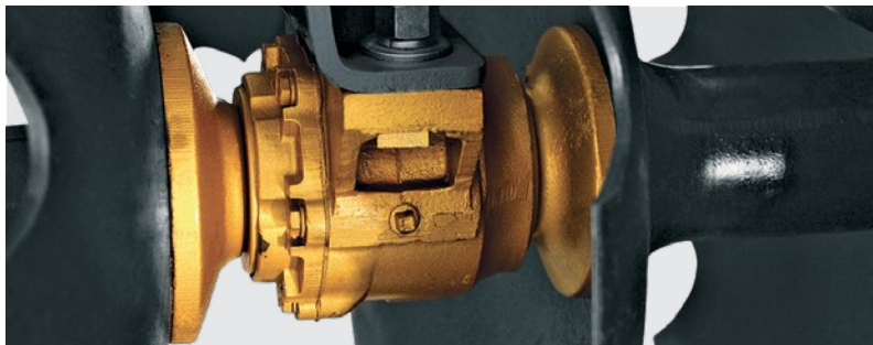
Mancais de rolamentos cônicos a banho de óleo com lubrificação permanente e vedação axial. Oil bath conical bearings with permanent lubrication and axial seal. Cojinetes de rodamientos cónicos en baño de aceite con lubricación permanente y sello axial.
