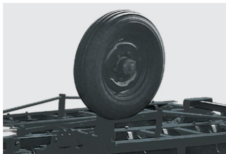
Rodeiro para transporte com pneu 600x16 (NVFP). Transport wheels 600x16 (NVFP). Rueda para transporte con neumático 600x16 (NVFP).
