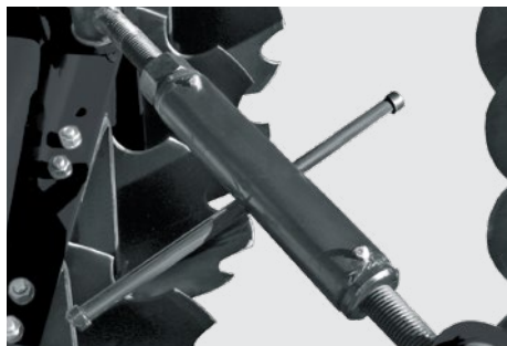
Regulamento de cruzamento de discos. Adjustment of the discs angle. Regulación de cruce de los discos.
