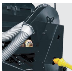
Turbina acionada por cardan nas versões: 4000/4500/5000/5500. Turbina acionada por motor hidráulico no sistema de fluxo contínuo do trator com vazão mínima de 30 litros. The turbine turns on by the PTO shaft on the versions: 4000/4500/5000/5500. Turbine driven by hydraulic motor with minimum flow of 30 liters. Turbina accionada a través de eje cardan en las versiones: 4000/4500/ 5000/5500. Turbina accionado por el motor hidráulico con flujo mínimo de 30 litros.
