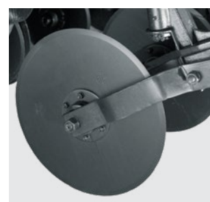
Discos de corte paralelos de 18" (para os modelos 4000, 4500, 5000 e 5500) e 20" desencontrados (para os modelos 6500 e 7500) com mola independente e regulagem de profundidade individual. Aligned cutter disc 18" (available for models 4000, 4500, 5000 and 5500), unaligned 20" (available for models 6500 and 7500) with independent spring and individual adjustment. Discos cortadores paralelos de 18" (para los modelos 4000, 4500, 5000 y 5500) y 20" desencontrados (para los modelos 6500 y 7500) con resorte independiente y regulación individual de la profundidad.
