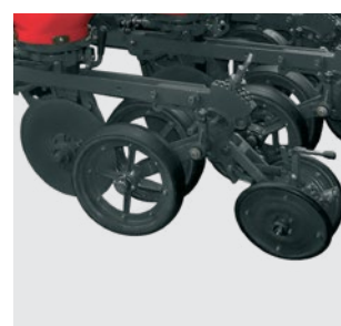
Rodas para controle de profundidade e compactação com regulagem manual. Wheels for depth control and compression with manual adjustments. Ruedas para control de profundidad y compactación con regulación manual.
