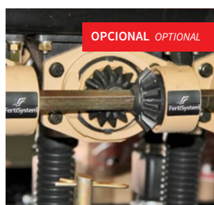
Conductor de adubo sistema Fertisystem transversal. Fertisystem fertilizer metering. Conductor de abono sistema Fertisystem transversal.
