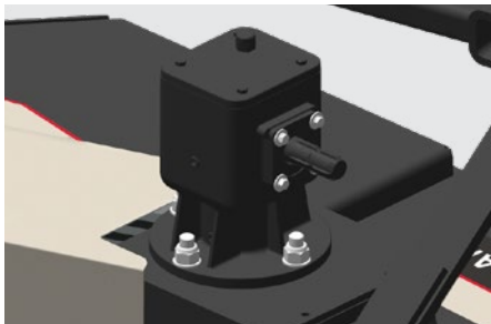
Caixa multiplicadora de velocidade de giro livre. Free-rotation gearbox. Caja multiplicadora de velocidad de giro libre.
