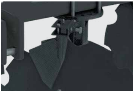
Limpadores de discos com regulagem.
