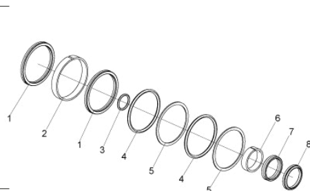
Kit De Sellado LENIORS
