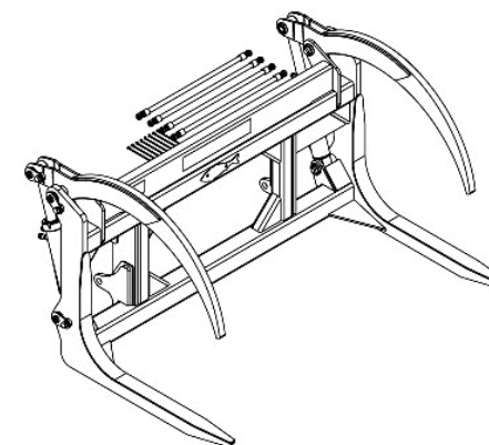
Garfo de Tora 5304010012-8 Vide página 38
