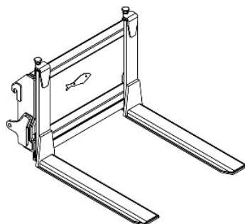
Garfo Pallet 5304010011-0 Vide página 36
