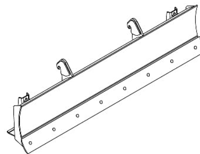
Lâmina 2400mm - 5340010028-0 2600mm - 5340010037-0 Vide página 44
