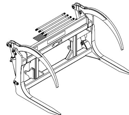
Garfo de Tora 5304010012-8 Vide página 43
