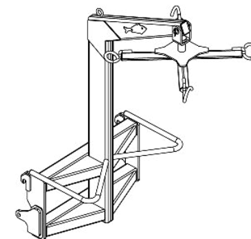
Guincho 2547260205-8 Vide página 44
