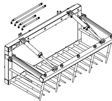
Garfo de Silagem 2547260502-2 Vide página 42
