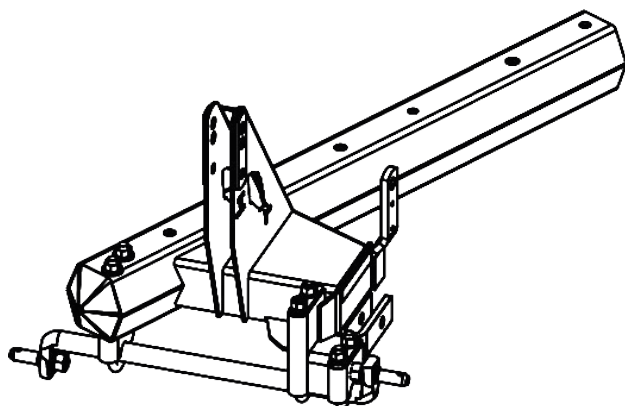
ARMAZÓN COMPLETO PARA LA EXPORTACIÓN AF 03 DISCOS
