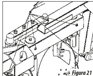
Soporte Inferior de la Rueda de Guía, Tornillos del Soporte y Bujes Inferior y Superior
