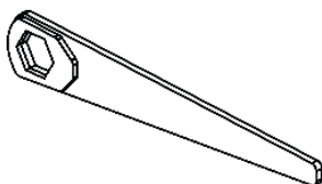
LLAVE P/ TUERCA HEXAGONAL DE 1 5/8"
