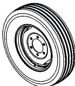
NEUMÁTICOS 650 X 16 8 LONAS USAR 54 LBS/POL 2
