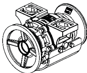
MANCAL AXIAL CON PROTECCIÓN
