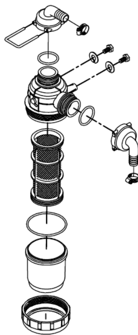
FILTRO DE SUCCIÓN
