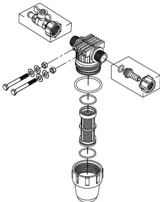
FILTRO DE LÍNEA
