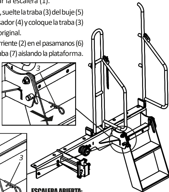
ESCALERA ABIERTA: POSICIÓN PARA EL SUMINISTRO O MANTENIMIENTO DE LOS TANQUES
