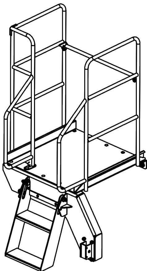
PLATAFORMA DERECHA COMPLETA PARA FC 600 SIEMBRA DOBLE ALTERNADA
