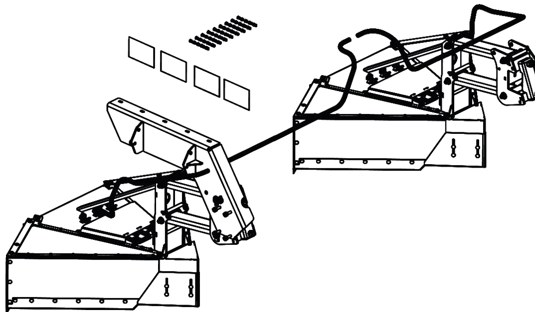
KIT ACCESORIOS PARA ADAPTACIÓN ESPACIADO DE SIEMBRA DOBLE ALTERNADA
