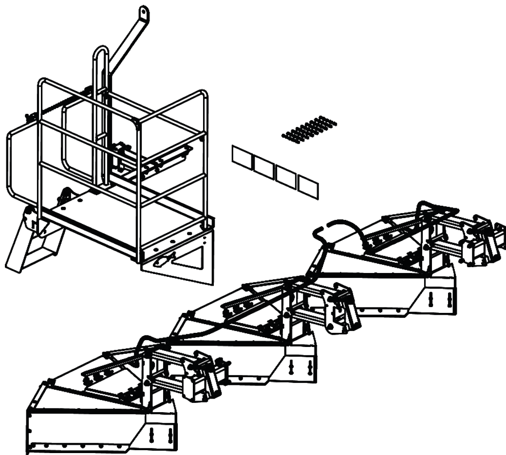
KIT ACCESORIOS PARA ADAPTACIÓN ESPACIADO DE SIEMBRA SIMÉTRICA DE 1,4 A 1,5 METROS
