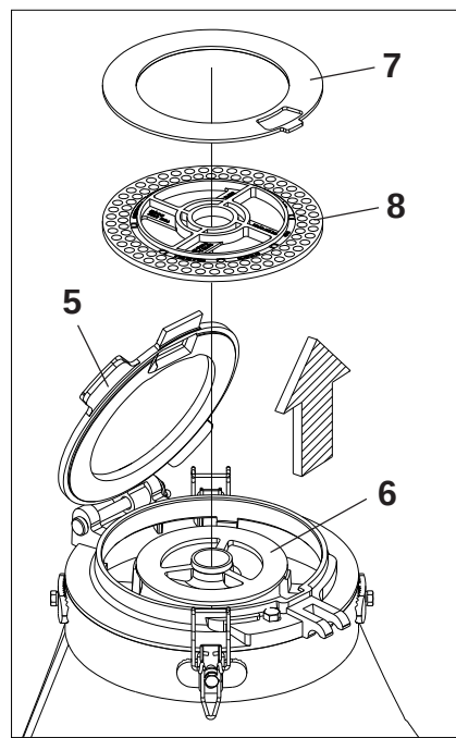
Detalle "F"
