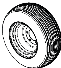
NEUMÁTICO 11 X 15 - BL 10 LONAS NVCR 48 A 56 DISCOS (ESPACIAMIENTO 175 MM) NVCR 42 A 64 DISCOS (ESPACIAMIENTO 200 MM)
