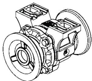
COJINETE DE GRASA SIN PROTECCIÓN ESPACIAMIENTO 175 MM Y 200 MM NVCR 28 A 56 DISCOS
