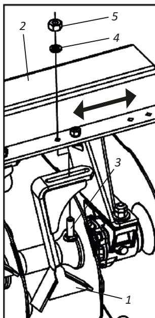
NVCR 60 Y 64 DISCOS ESPACIAMIENTO DE 200 MM
