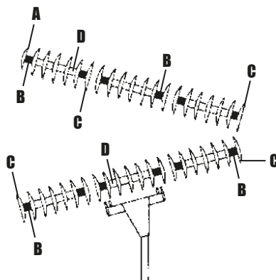
NV/NVP 42 DISCOS ESPACIADO 175 Y 200 MM
