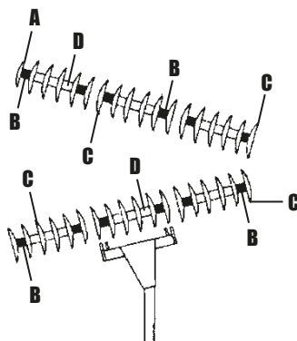
NV/NVP 36 DISCOS ESPACIADO 200 MM
