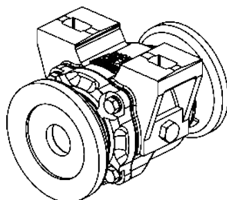
COJINETE CON ACEITE Y SIN PROTECCIÓN ESPACIAMIENTO 175 Y 200 MM
