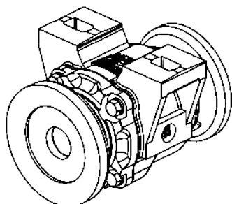
COJINETE CON GRASA SIN PROTECCIÓN ESPACIAMIENTO 175 Y 200 MM
