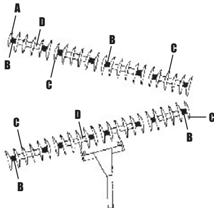
NV/NVP 48 DISCOS ESPACIADO 200 MM
