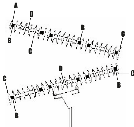
NV/NVP 48 DISCOS ESPACIADO 175 MM
