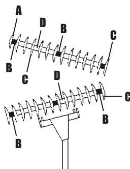
NV/NVP 28 DISCOS ESPACIADO 175 MM
