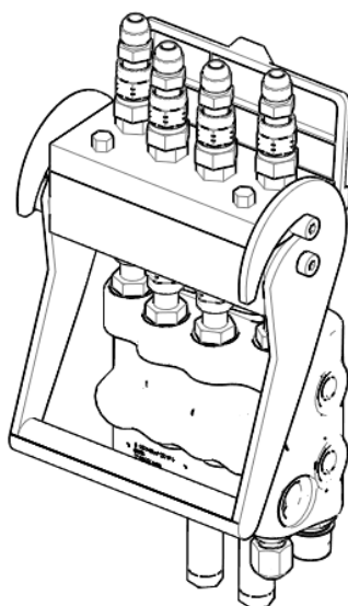
SISTEMA DE ENGANCHE HIDRÁULICO MULTIFASTER
