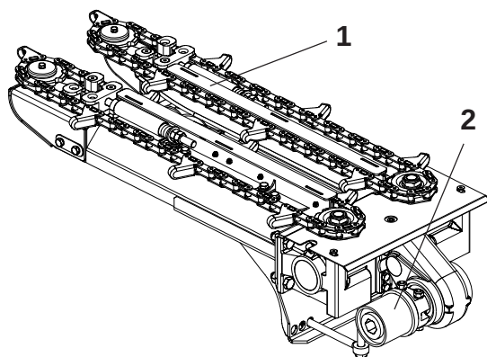
Línea de Cosecha (1) con Limitador de Torque (2)
