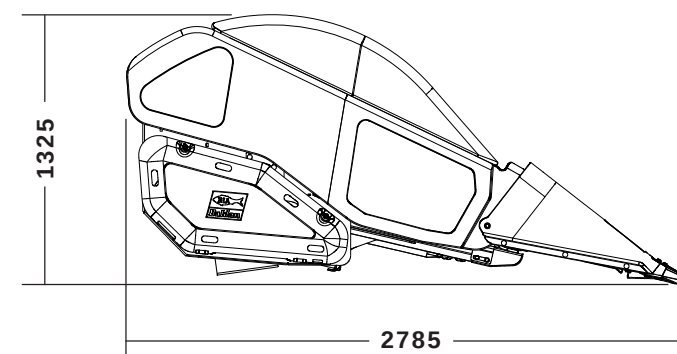
Vista Lateral de la POTENZA
