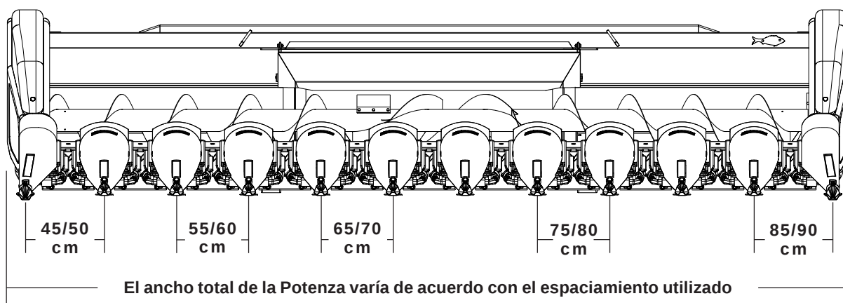
Vista Frontal de la POTENZA
