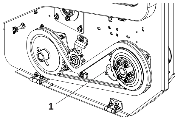
Engranaje Lateral (1) con Embrague
