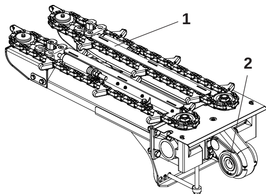
Línea de Cosecha (1) sin Limitador de Torque (2)
