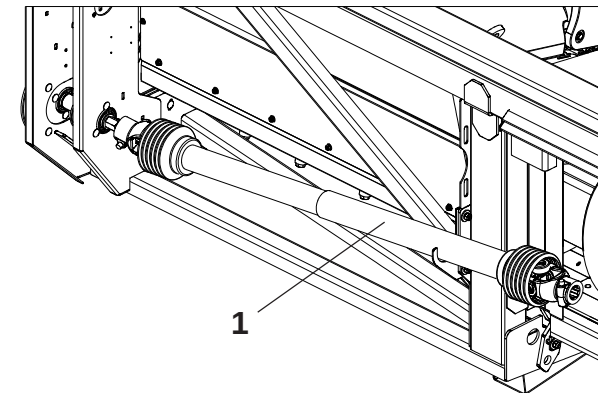
Eje Cardan (1) sin Embrague
