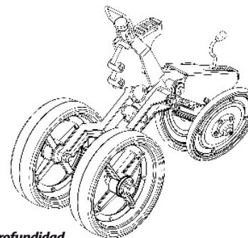
Carro c/ rueda de profundidad oscilante y p/ plantio de algodón y rueda en "V" completo
