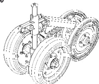
Carro c/ rueda de profundidad fija y rueda en "V" completo
