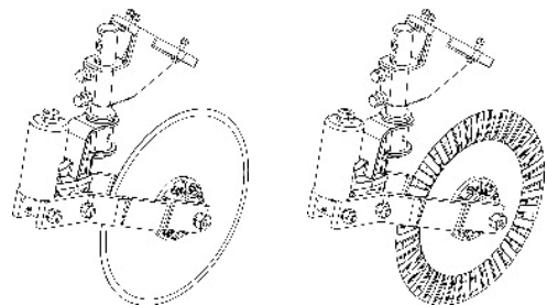
Soporte c/ disco de corte liso de 18" y 20" y disco estriado de "18" - 4000 a 5500
