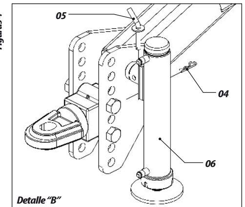
Detalle "B"
