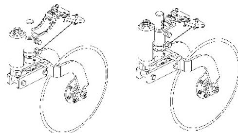
Soporte mayor y menor c/ disco de corte liso de 20" - 6500 y 7500
