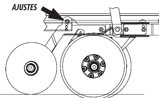
Rueda Compactadora para Doble Disco
