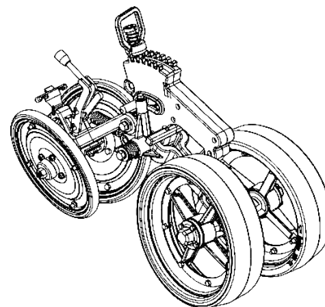
Carro c/ Rueda de Profundidad p/ Rueda Involucrando Disco y Rueda en "V" Cpl s/ Batidor - Código: 51240103625
