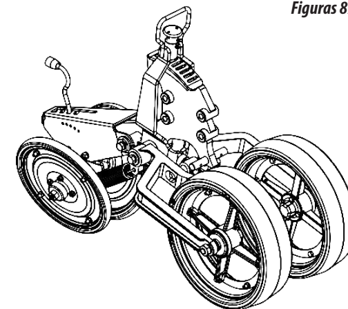
Carro c/ Ruda de Profundidad p/ Rueda Involucrando Disco y Rueda en "V" Cpl c/ Batidor - Código: 51240103609
