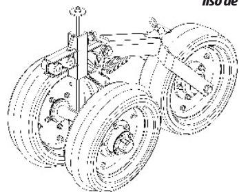
Carro completo de la rueda compactadora lisa, concava y convexa
