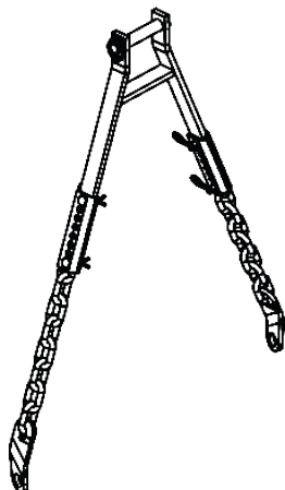
ENGANCHE LIMITADOR DE ALTURA ( MODELO RP )
