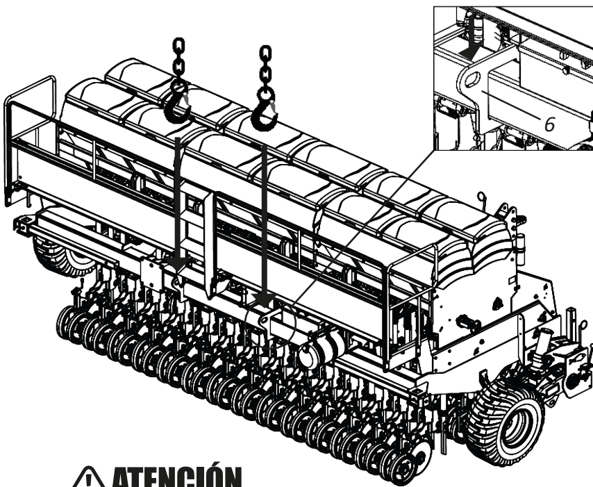
ENGANCHES TRASEROS
