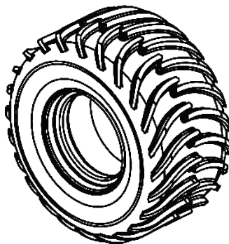
NEUMÁTICOS 500/60 - 22.5 16 PR TR-08 TL USAR: 48 LBS/POL 2
