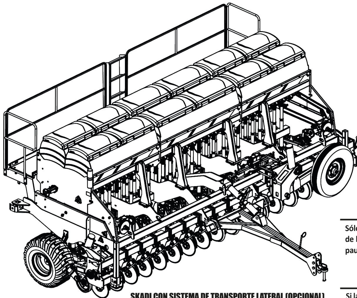
SKADI CON SISTEMA DE TRANSPORTE LATERAL (OPCIONAL) LISTA PARA EL TRABAJO
