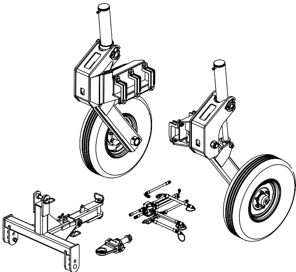
SISTEMA DE TRANSPORTE LATERAL SKADI 5000 / 6000 / 7000
