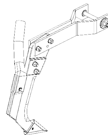
SURCADOR DEL ABONO CON DEFLECTOR
