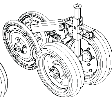
Carrito de la rueda de profundidad y rueda "V" Código: 5124010050-2
