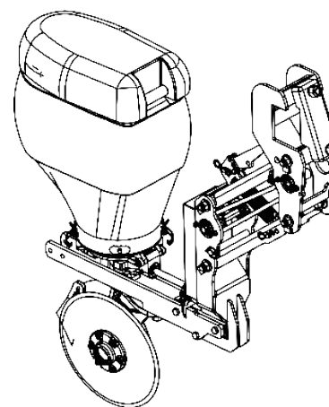
Línea pantográfica menor derecha Baldan (2019)
