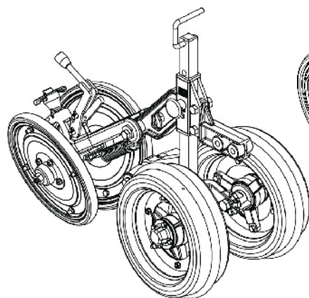
Carrito de la rueda de profundidad Excentrica Oscilante y rueda "V" Código: 5124010557-1
