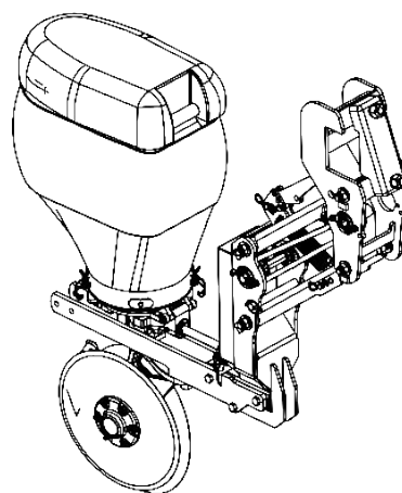
Línea pantográfica menor Izquierda Baldan (2019)
