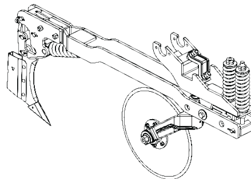
Carrinho maior sulcador automático Código: 5124010610-1
