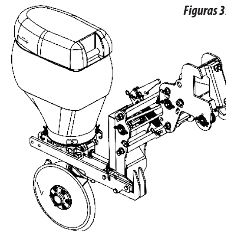
Línea pantográfica mayor izquierda Baldan (2019)
