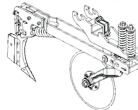
Carrito menor surcador automático Código: 5124010609-8
