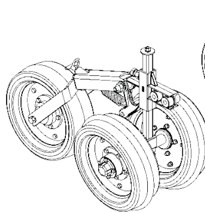
Carrito de la rueda compactadora lisa Código: 5124010113-4
