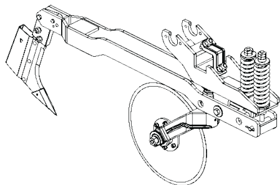
Carrito mayor c/ surcador Código: 5124010531-8
