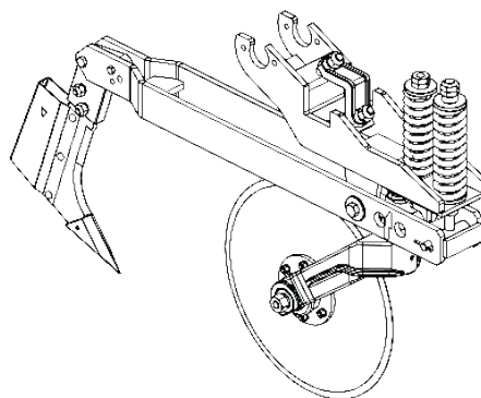
Carrito menor c/ surcador cpl Código: 5124010530-0
