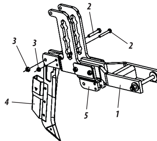
Sistema para paja densa
