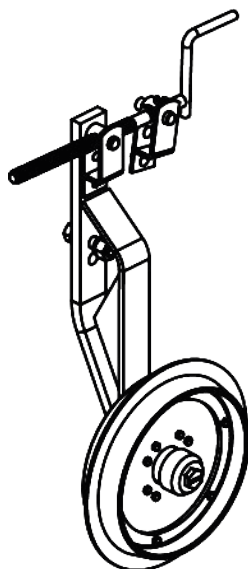
RODA DE PROFUNDIDADE COM MANIVELA AF/AFL
