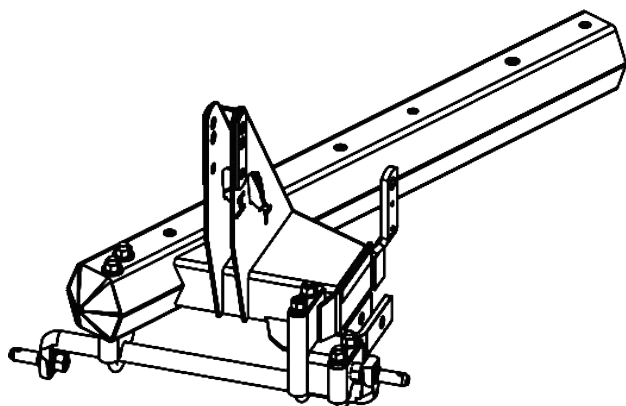
ARMAÇÃO COMPLETA PARA EXPORTAÇÃO AF 03 DISCOS
