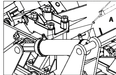
Figura 24 - Pistão Hidráulico
