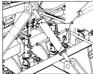
Figura 27 - Regulador do cabeçalho
