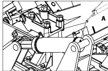
Figura 24 - Pistão Hidráulico
