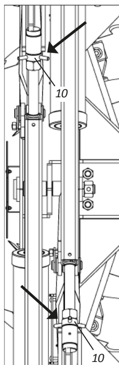
DETALHE "A"
