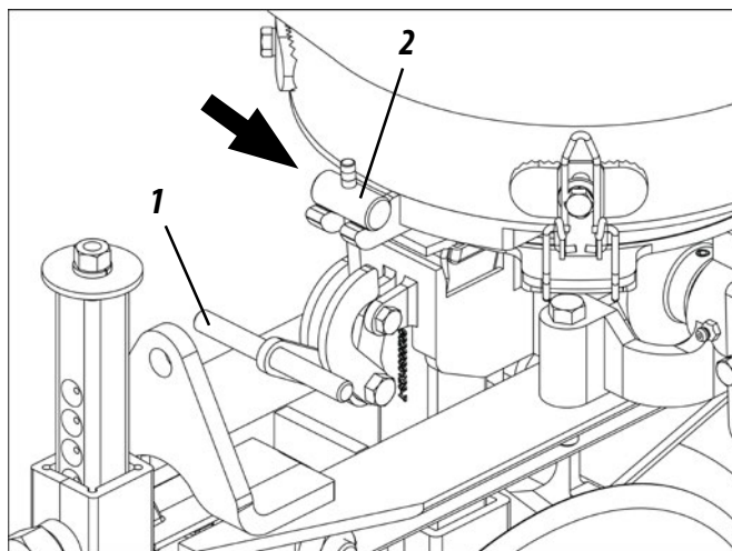
Detalhe "A"
