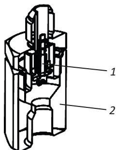
VISTA INTERNA DO NIPLE
