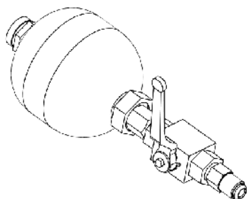
ACUMULADOR COM REGISTRO DE ESFERA
