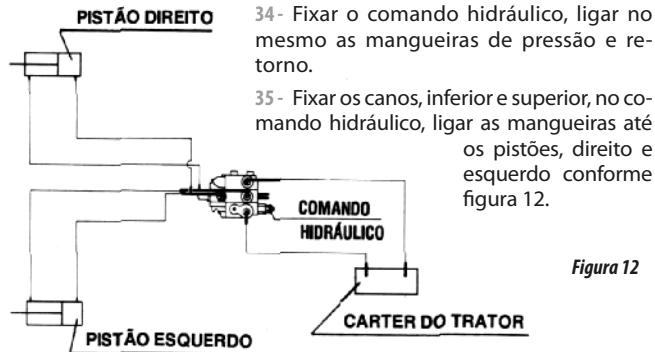
Esquema hidráulico BT, ligado na saída de pressão e retorno da carcaça do trator.
