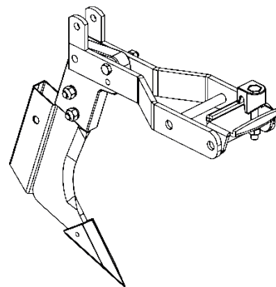
SULCADOR DA HASTE COM SUPOORTE COMPLETO
