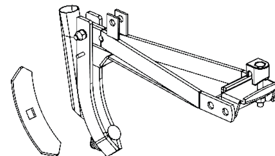
SUPOORTE COM BICO RISCADOR PARA ADUBAÇÃO PROFUNDA
