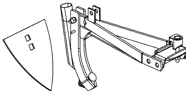
SUPOORTE COM BICO SULCADOR PARA PLANTIO DE MILHO
