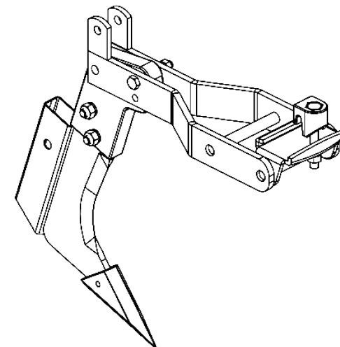
SULCADOR PONTIAGUDO COM PONTA REMOVÍVEL PARA ADUBO
