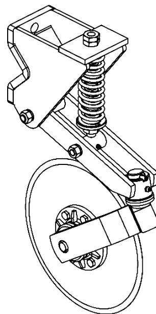
DISCO DE CORTE (LISO OU ESTRIADO)
