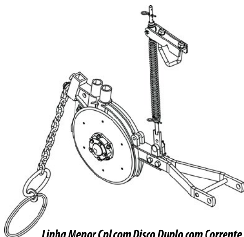
Linha Menor Cpl com Disco Duplo com Corrente Código: 2517011506-9
