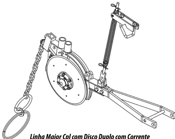
Linha Maior Cpl com Disco Duplo com Corrente Código: 2517011507-7
