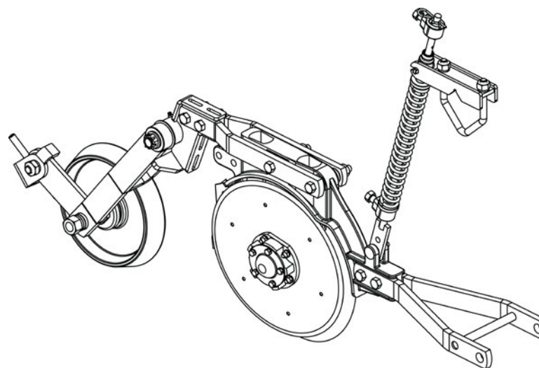
Linha Menor Esquerda c/ Roda Ferro (Descentrado) Código: 2517011741-0
