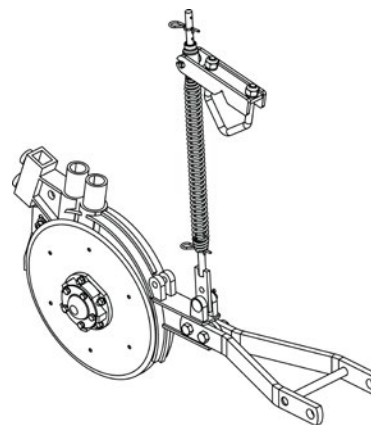
Linha Menor Cpl com Disco Duplo sem Corrente Código: 5124010568-7
