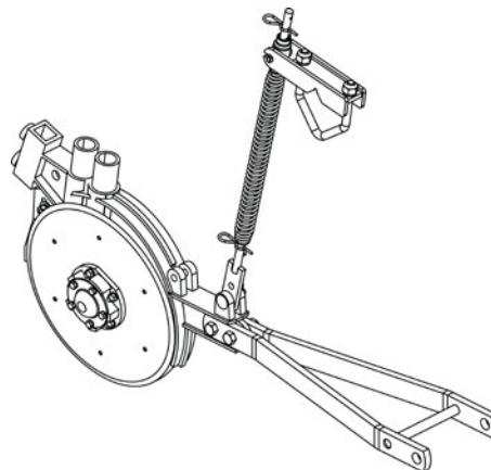
Linha Maior Cpl com Disco Duplo sem Corrente Código: 5124010570-9
