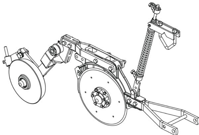
Linha Menor Direita c/ Roda Ferro (Descentrado) Código: 2517011740-1
