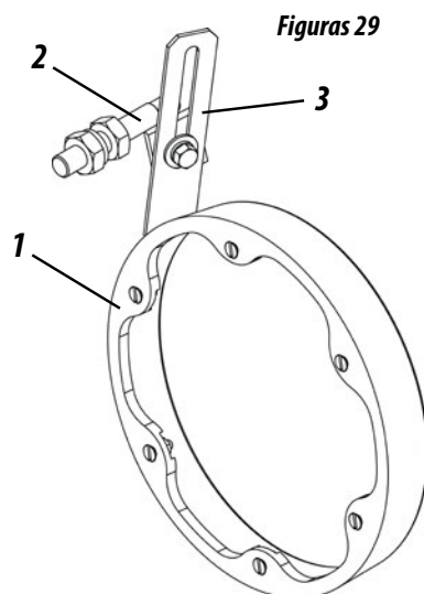
Friso de Profundidade Direito Cpl Código: 5288010047-5
