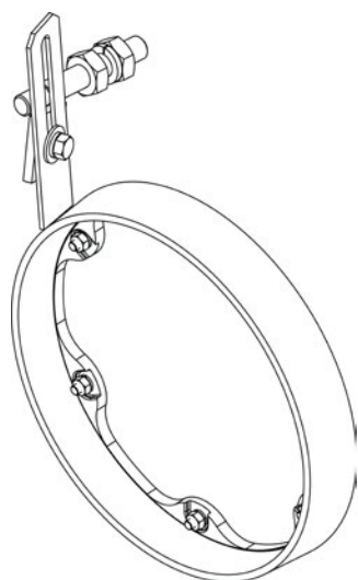
Friso de Profundidade Esquerdo Cpl Código: 5288010046-7
