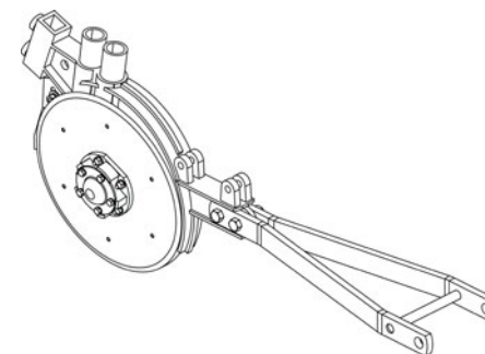
Carrinho Montado Maior Código: 5124010571-7
