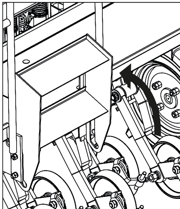
POSIÇÃO FECHADA: PARA TRABALHO OU TRANSPORTE
