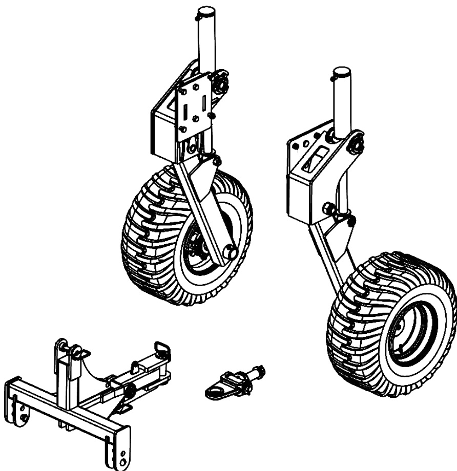
SISTEMA DE TRANSPORTE LATERAL SKADI 4000 / 5000 / 6000 / 7000 / 8000 / 9000
