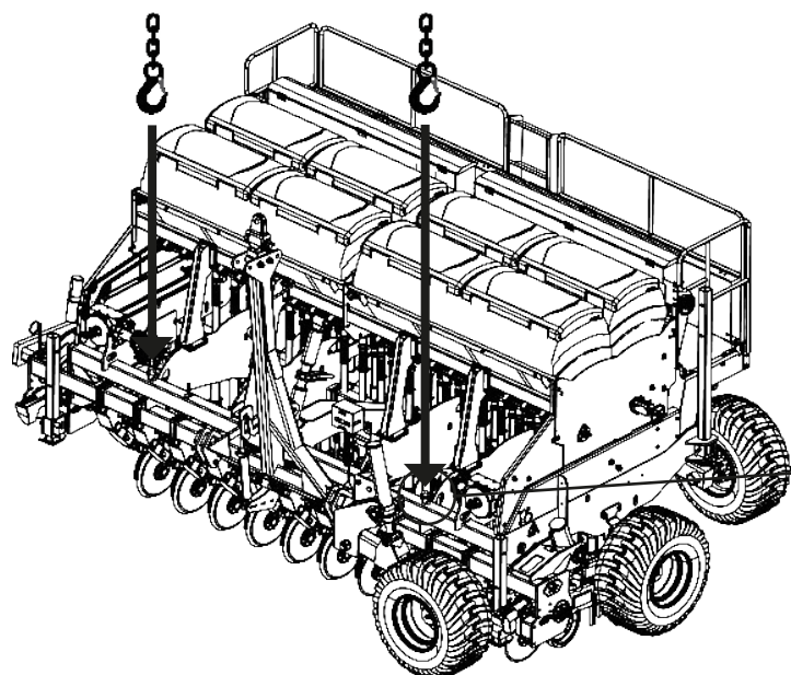
ENGATES DIANTEIROS
