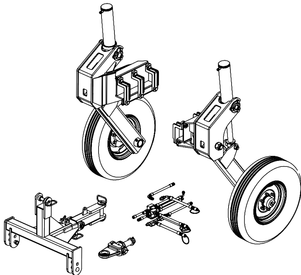
SISTEMA DE TRANSPORTE LATERAL SKADI 5000 / 6000
