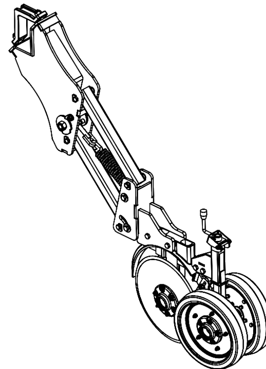
LINHA TRASEIRA ESQUERDA C/ DISCO DUPLO ADUBO/SEMENTE C/ REGULADOR DE PROFUNDIDADE ( RODA LARGA )
