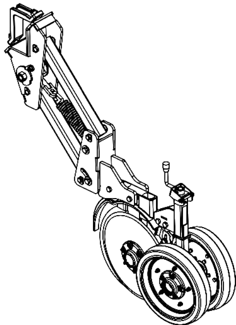
LINHA DIANTEIRA DIREITA C/ DISCO DUPLO ADUBO/SEMENTE C/ REGULADOR DE PROFUNDIDADE ( RODA LARGA )
