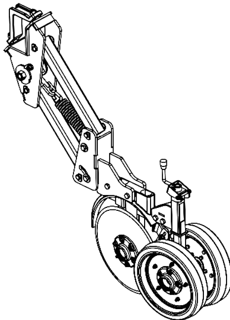
LINHA DIANTEIRA ESQUERDA C/ DISCO DUPLO ADUBO/SEMENTE C/ REGULADOR DE PROFUNDIDADE ( RODA LARGA )
