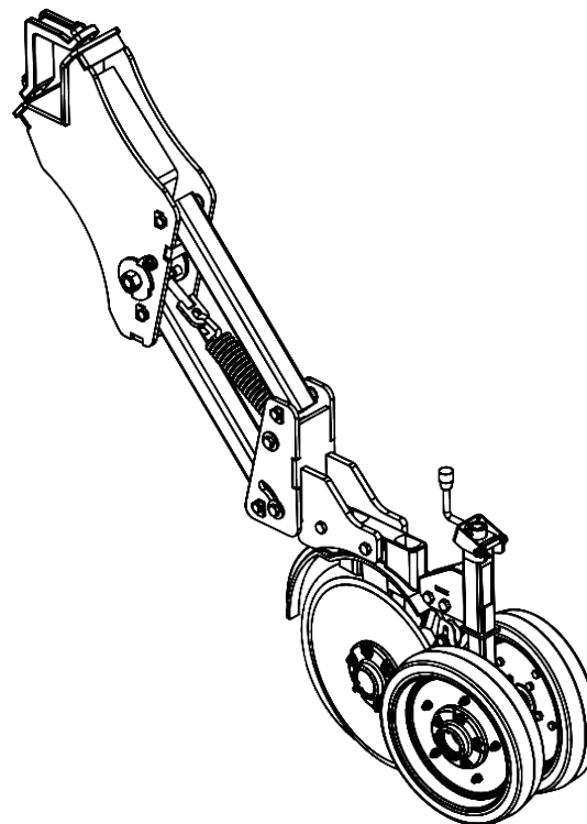
LINHA TRASEIRA DIREITA C/ DISCO DUPLO ADUBO/SEMENTE C/ REGULADOR DE PROFUNDIDADE ( RODA LARGA )
