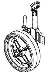
12 RODA DE REG. DE PROF. C/SUPOORTE
