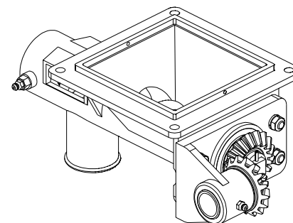
CONDUTOR TRANSVERSAL
