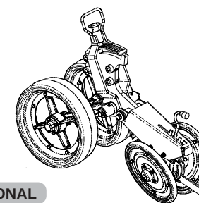
CARRINHO C/ RODA DE PROFUNDIDADE EXCÊNTRICA / OSCILANTE E RODA EM "V"
