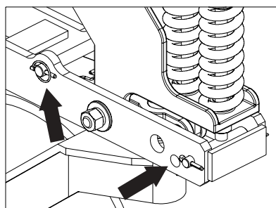
Sistema “Pula-Obstáculo” Ativado
