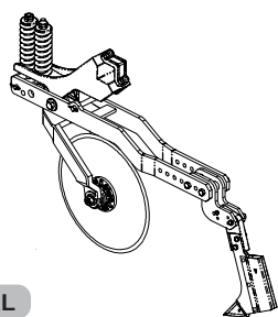
CARRINHO MAIOR E MENOR C/ SULCADOR DO ADUBO
