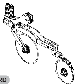
CARRINHO MAIOR E MENOR C/ SULCADOR DESARME E REARME AUTOMÁTICO
