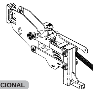
CARRINHO C/ RODA DE PROFUNDIDADE EXCÊNTRICA / OSCILANTE E RODA EM "V"
