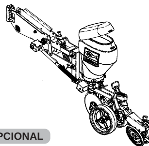
CARRINHO PANTOGRÁFICO MAIOR E MENOR DIREITO E ESQUERDO
