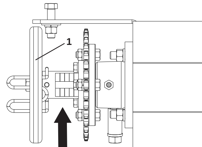
Detalhe “A”
