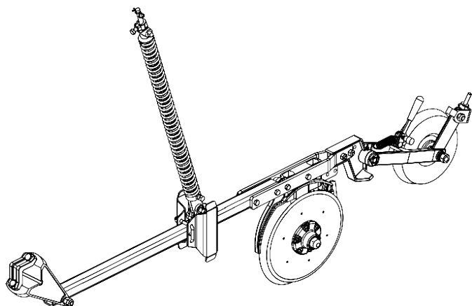
Linha direita maior c/ roda compactadora de ferro pesada
