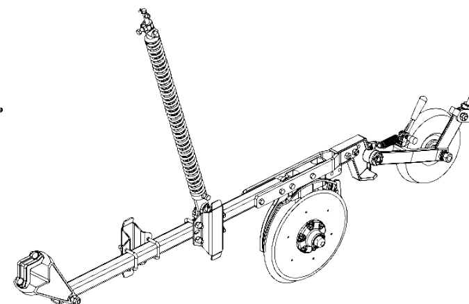
Linha lateral direita maior c/ roda compactadora de ferro pesada
