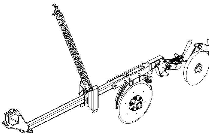
Linha esquerda maior c/ roda compactadora de ferro pesada
