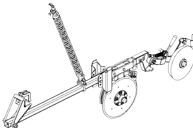
Linha esquerda menor c/ roda compactadora de ferro pesada
