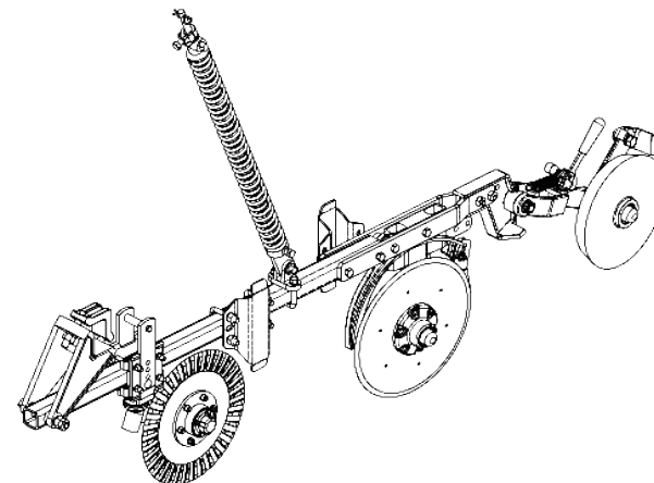
Linha direita lateral esquerda menor c/ disco de corte estriado c/ roda compactadora de ferro pesada
