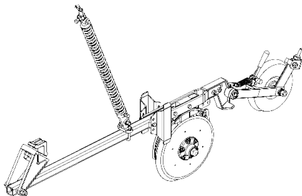
Linha direita menor c/ roda compactadora de ferro pesada
