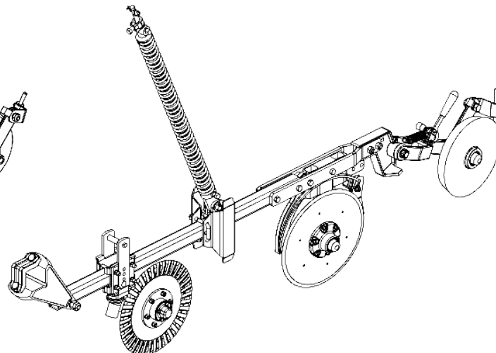
Linha esquerda menor c/ disco de corte estriado c/ roda compactadora de ferro pesada
