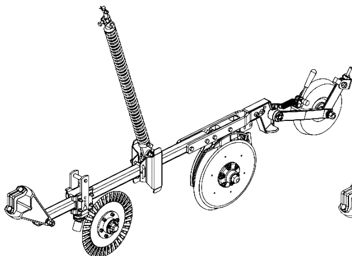
Linha direita menor c/ disco de corte estriado c/ roda compactadora de ferro pesada
