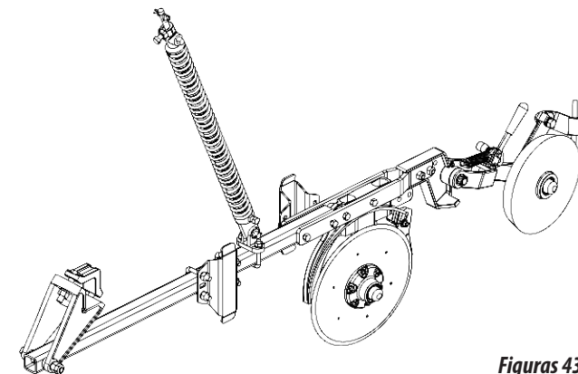
Linha lateral esquerda menor c/ roda compactadora de ferro pesada
