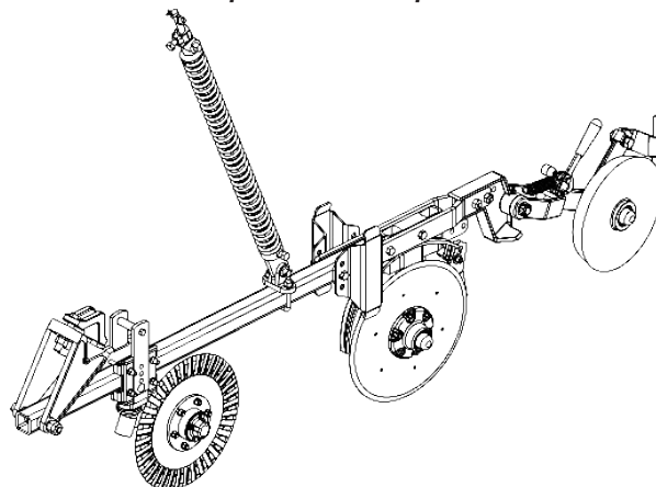
Linha esquerda menor c/ disco de corte estriado c/ roda compactadora de ferro pesada
